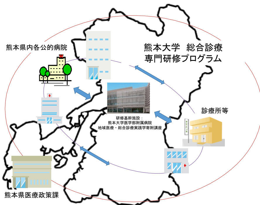
図1：研修体制
